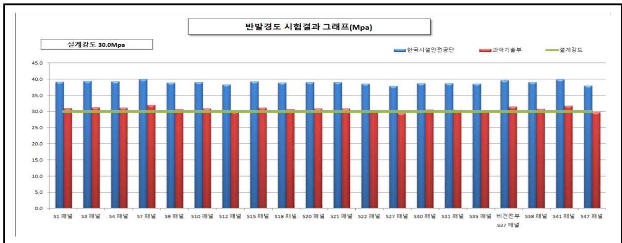
【그림 8.4.2】 반발경도시험 측정결과
