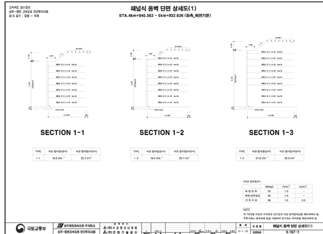
【그림 8.1.4】 단면도
