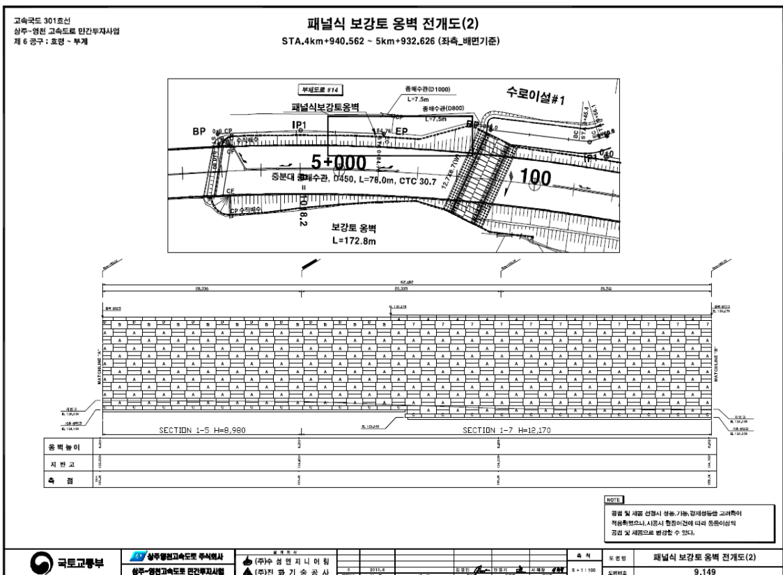
【그림 8.1.3】 전개도
