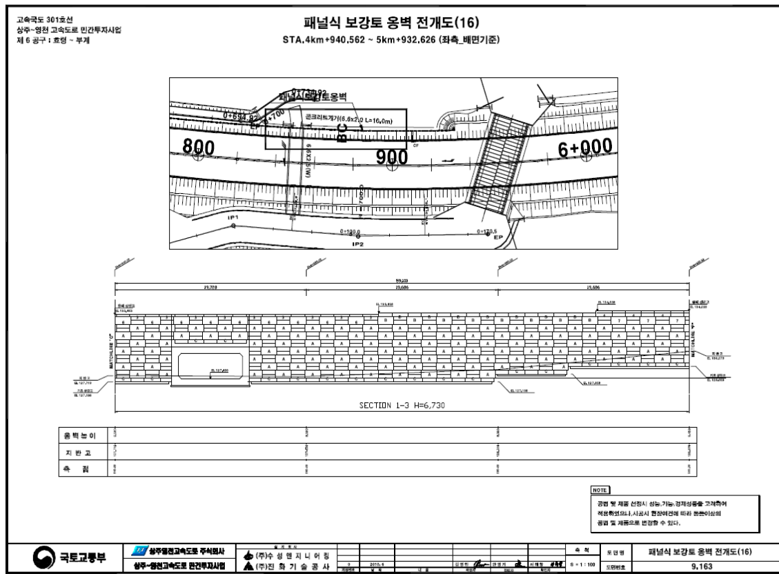
【그림 8.1.3】 전개도(계속)
