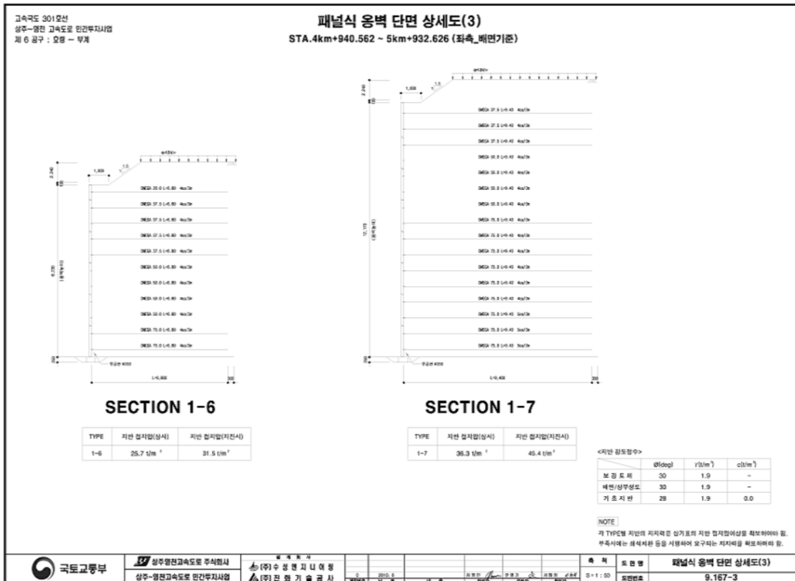
【그림 8.1.4】 단면도(계속)
